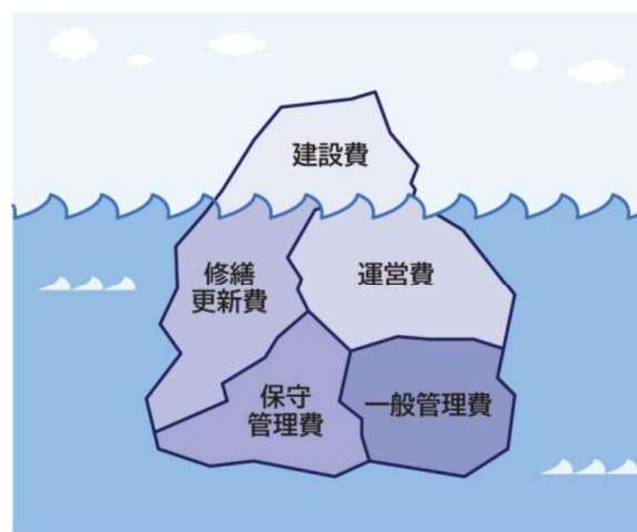
図 ライフサイクルコストの概念図
